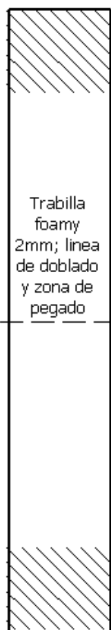
Soporte anilla; foamy 2 mm; línea de doblado y zona de pegado
